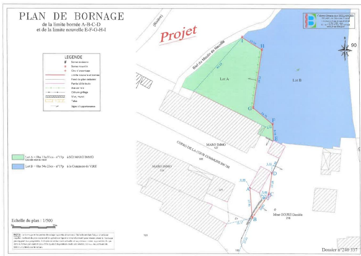
Figure 1 - Extrait du plan de bornage
